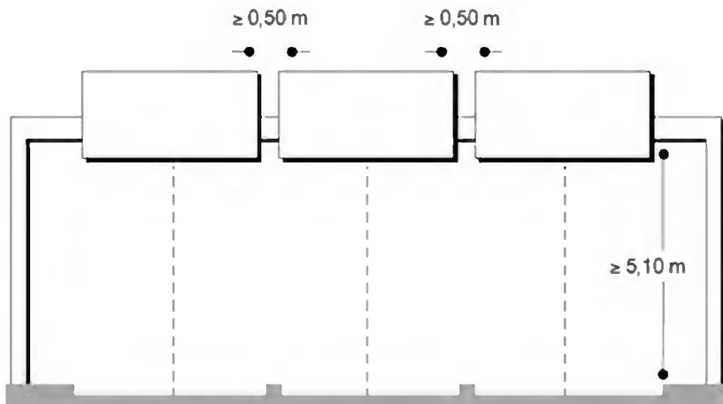
Installazione a portale su tre corsie
