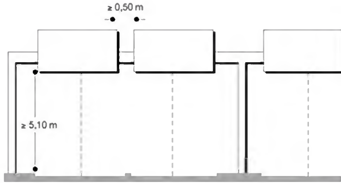
Installazione a portale con bandiera
