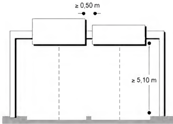
Installazione a portale su due corsie
