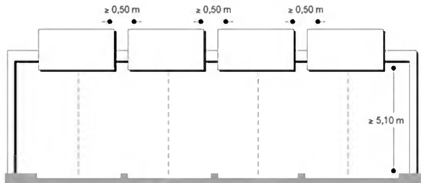
Installazione a portale su quattro corsie
